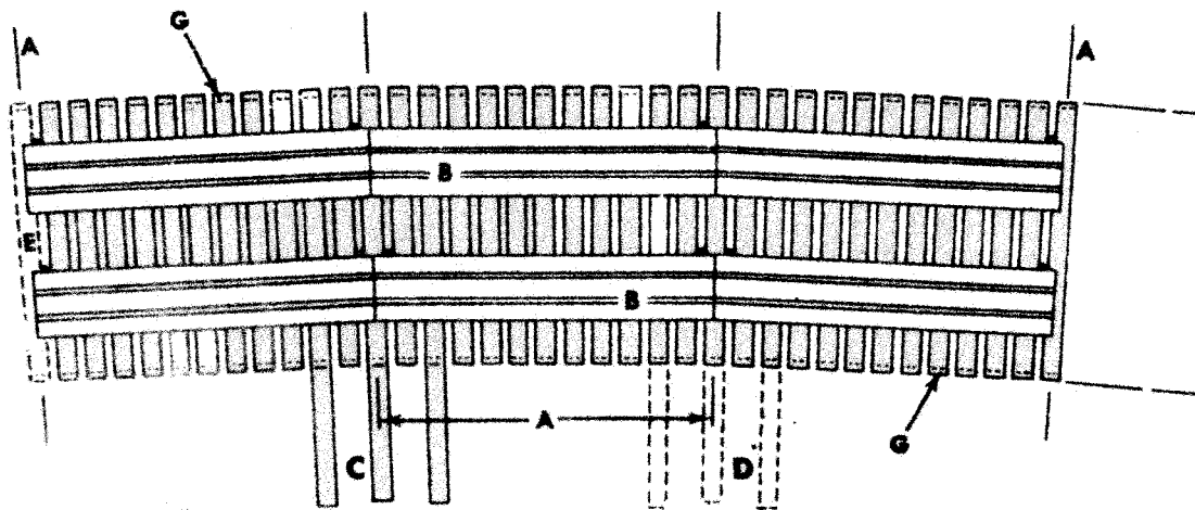
36" RADIUS
