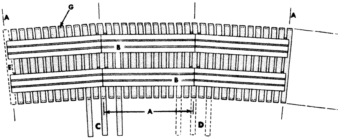
26" RADIUS
